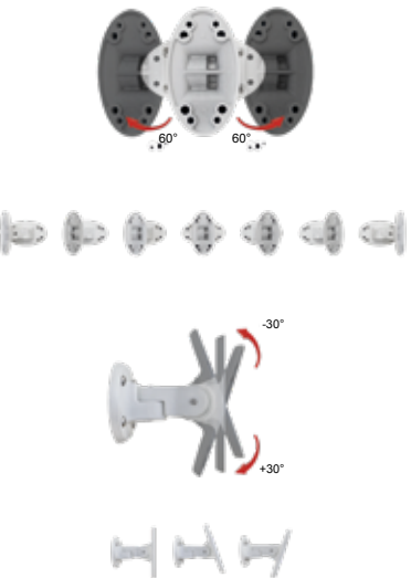
SUPPORTO PER IL FISSAGGIO A PARETE IN DOTAZIONE BRACKET FOR WALL MOUNTING INCLUDED
